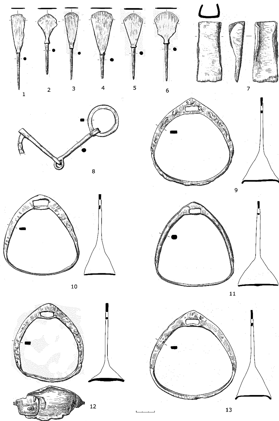
Рис.4. Могильник Ала-Тей 2. Объект 2. Предметы из железа. 1–6 – наконечники стрел; 7 – тесло; 8 – удила; 9–13 – стремена
